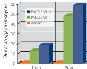
Сравнение ударостойкости Испытания проводились при 23°C в соответствии с ISO 6301/1 E50
