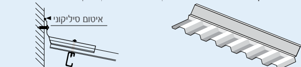
מפגש קיר-גג עליון | חתך רוחב דרך מפגש קיר-גג עליון
